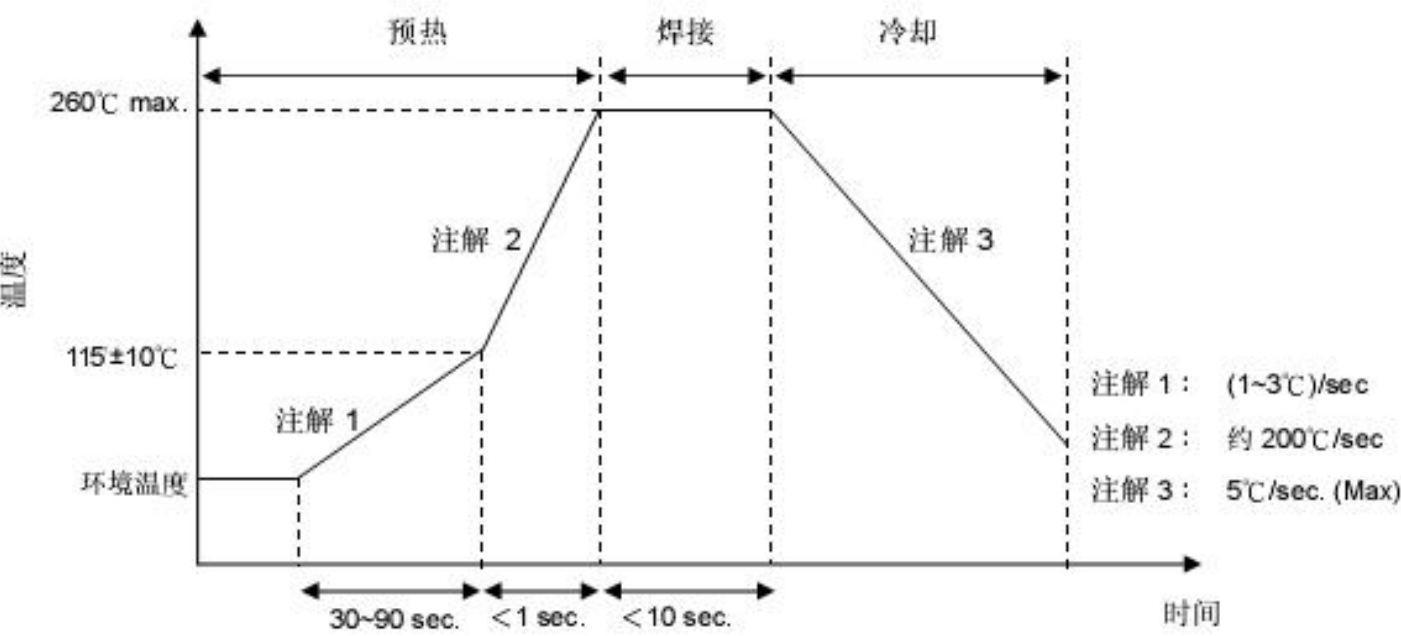
波峰焊曲线
